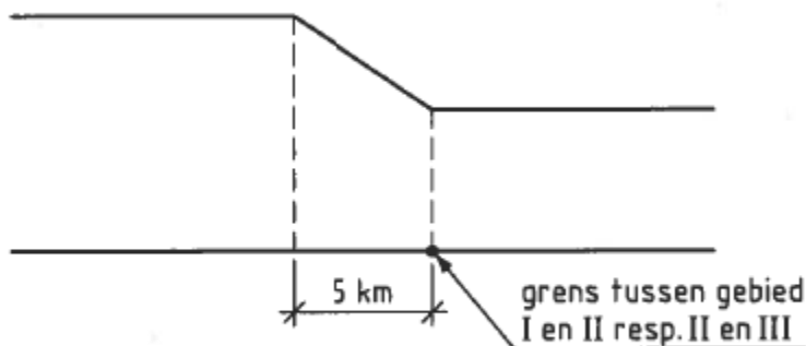
Figuur NB.2 — Overgangsg gebied tussen de windgebieden
