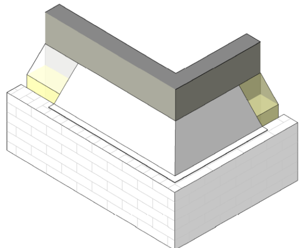
Afb. 47 Uitwendige hoek met spouwsteun
