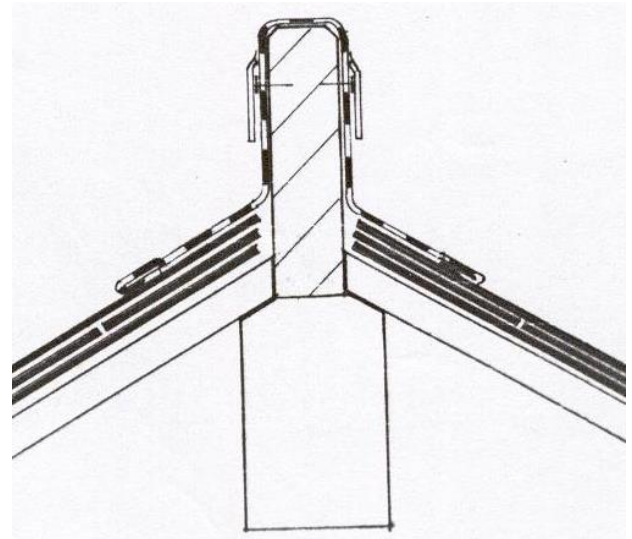
Afb. 53 I delig. Noklood
