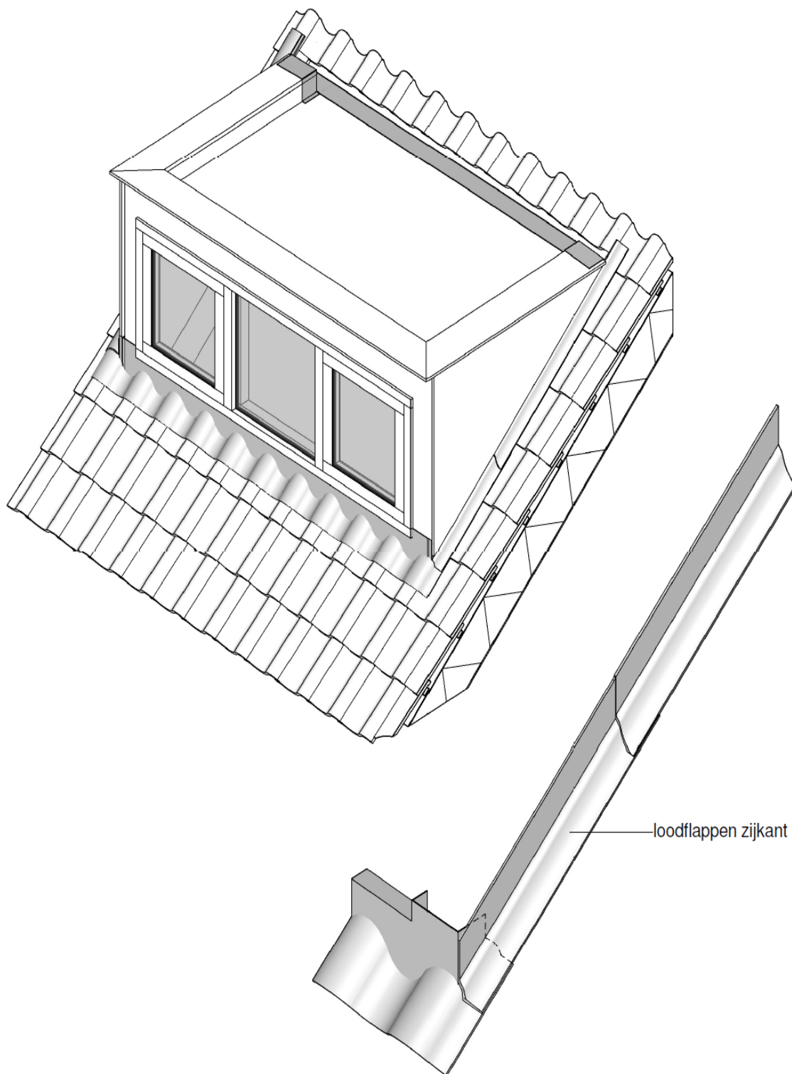
Afb. 41 ingedekte dakkapel
