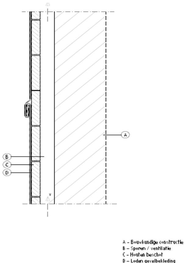
Afb. 3.3. Principe-constructie-opbouw on-geïsoleerde gevel
