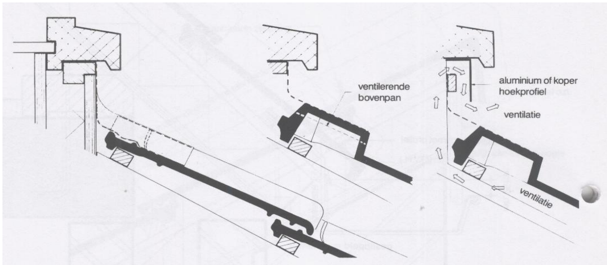
Afb. 48 3 verschillende onder aansluitingen: lood op pan, lood op bovenpan en lood op bovenpan geventileerd
