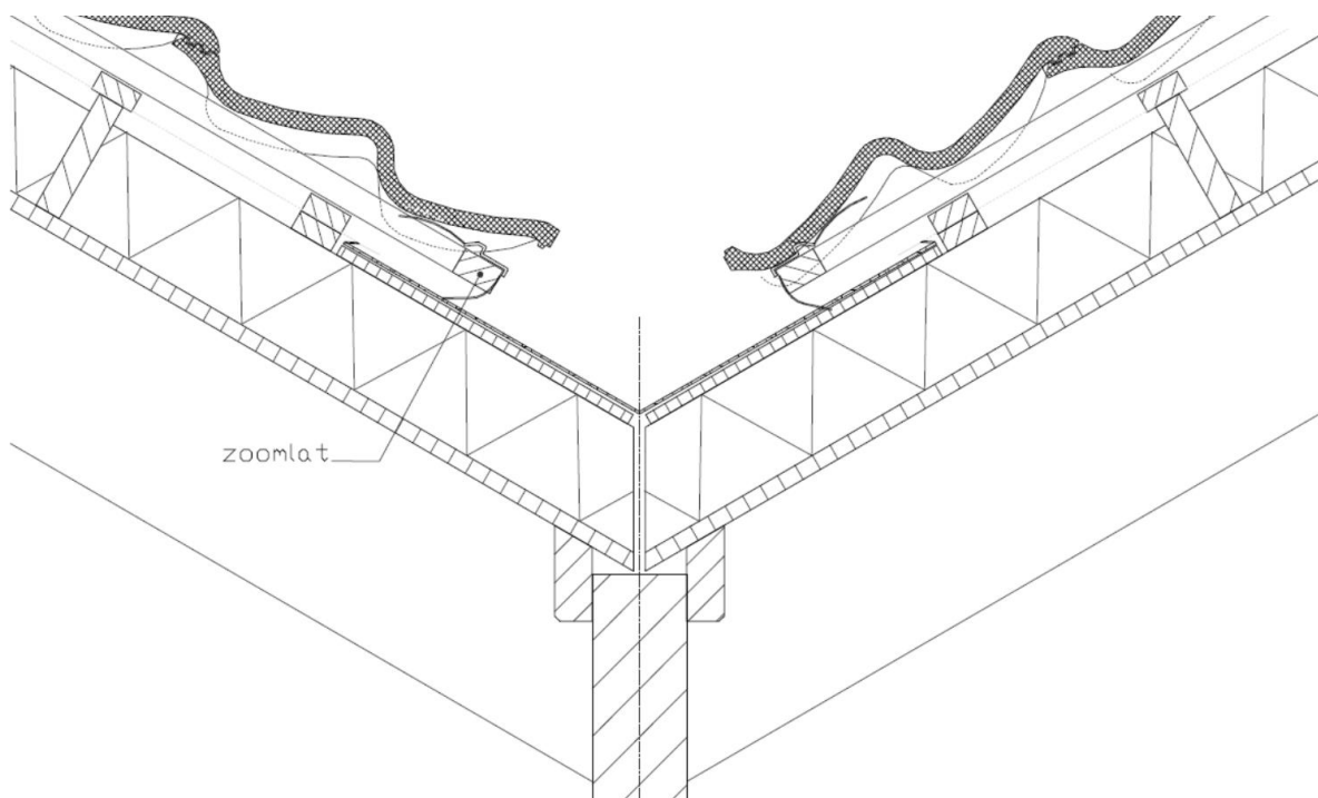
Afb. 8 Vlakke kilgoot volledig ondersteund
