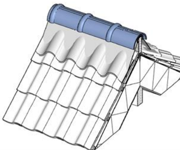
Afb. 56 Nok met ingedreven lood afgedekt met halfronde vorst
