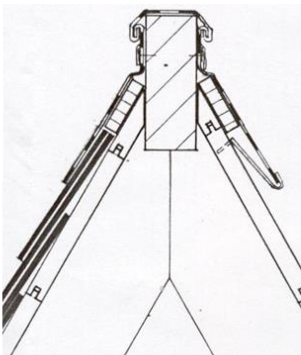
Afb. 55 3 dlg. Noklood
