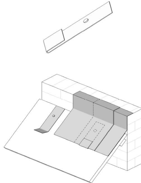
afb. 25 lood onder schoorsteen waarborg tegen opwaaien
