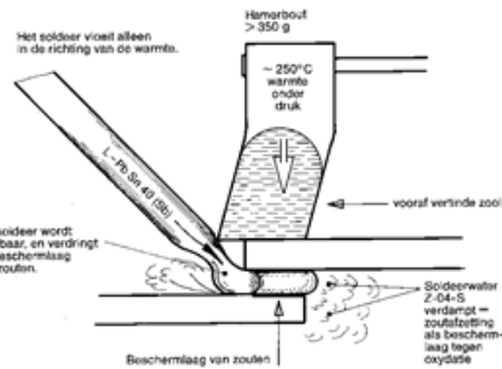
afb. 3 capillair bij solderen
