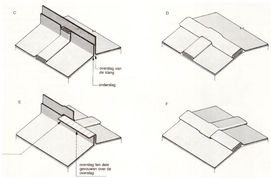
Afb. 21 felsuitvoering bij niet geventileerde nok
