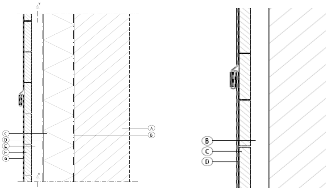
Afb. 39 Gevel bekleding in geïsoleerde en on- geïsoleerde uitvoering
