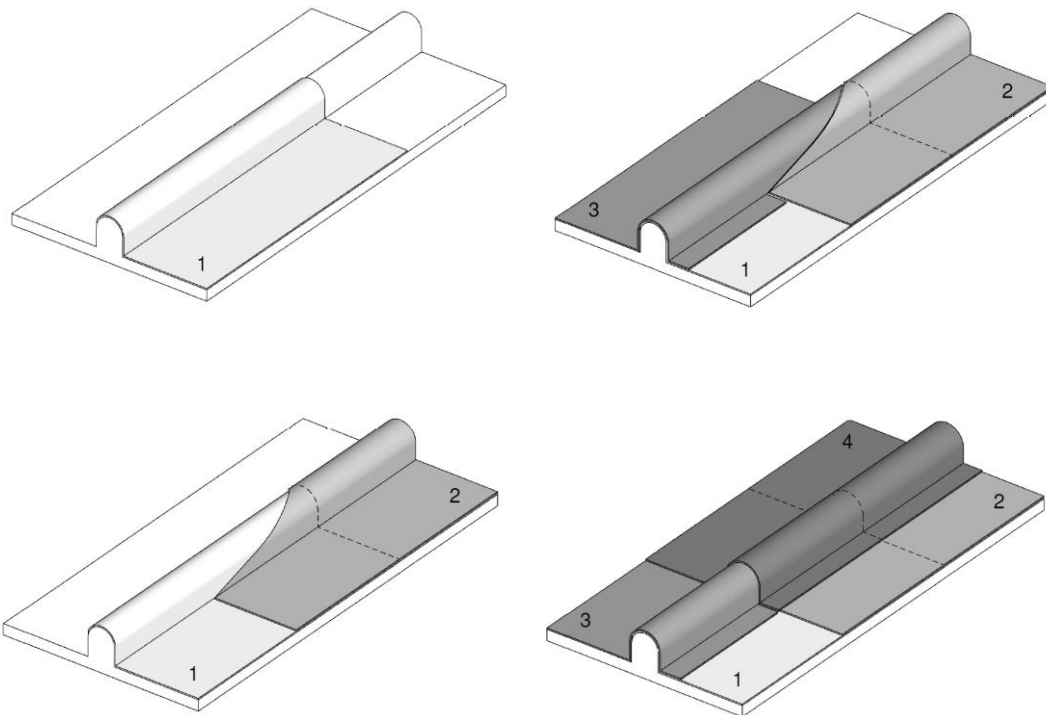
Afb 16 Overlappen verticaal en horizontaal roefbanen
