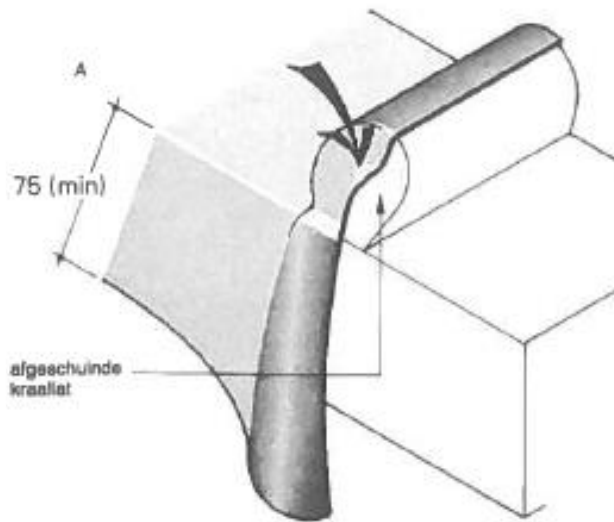
Afb. 18 c dakvoet uitvoering met roeflat afgeschuind
