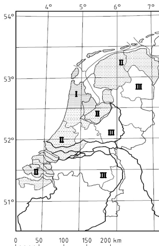
Afb. 57 Windgebieden in Nederland
