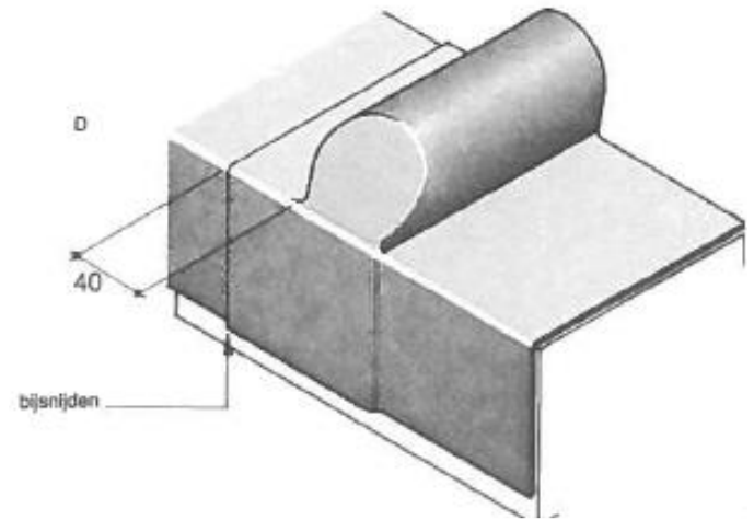
Afb. 18 d uitvoering dakvoet
