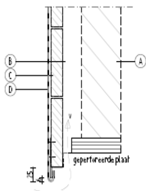
Afb. 31 enkele en dubbele fels uitvoering
