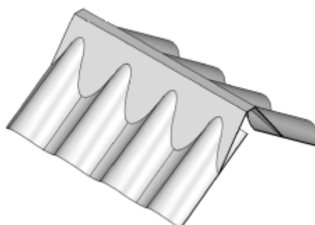
Afb. 58 Lood op nok zonder vorst
