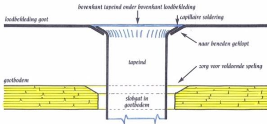
Afb. 2 uitloop in goot met speling
