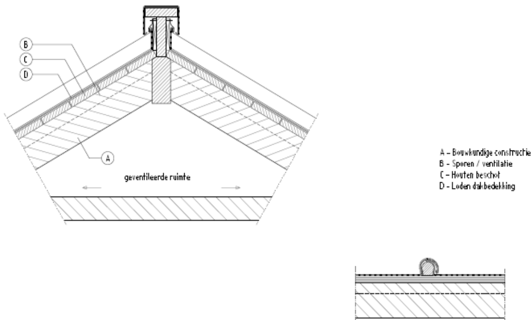
Afb. 3.3. Principe-constructie-opbouw ongeïsoleerd dak
