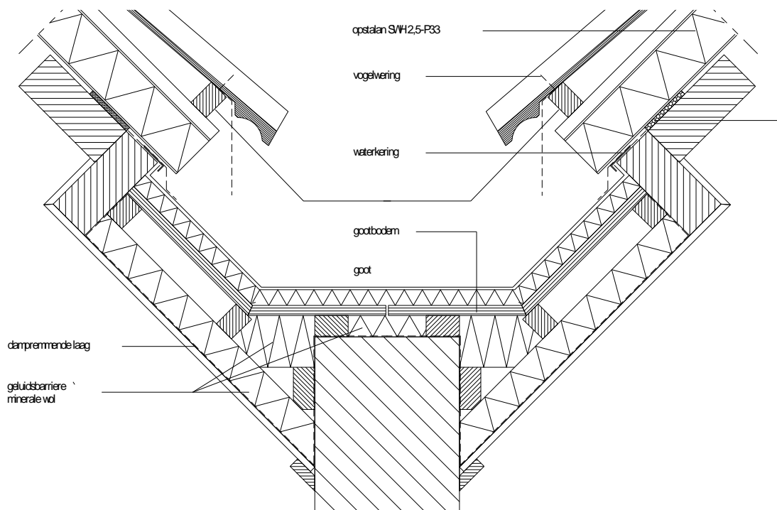
afb. 11 zakgoot in geïsoleerd dak volledig ondersteund
