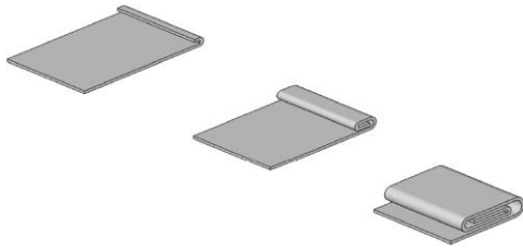
Afb 42 Opgerolde loodprop
