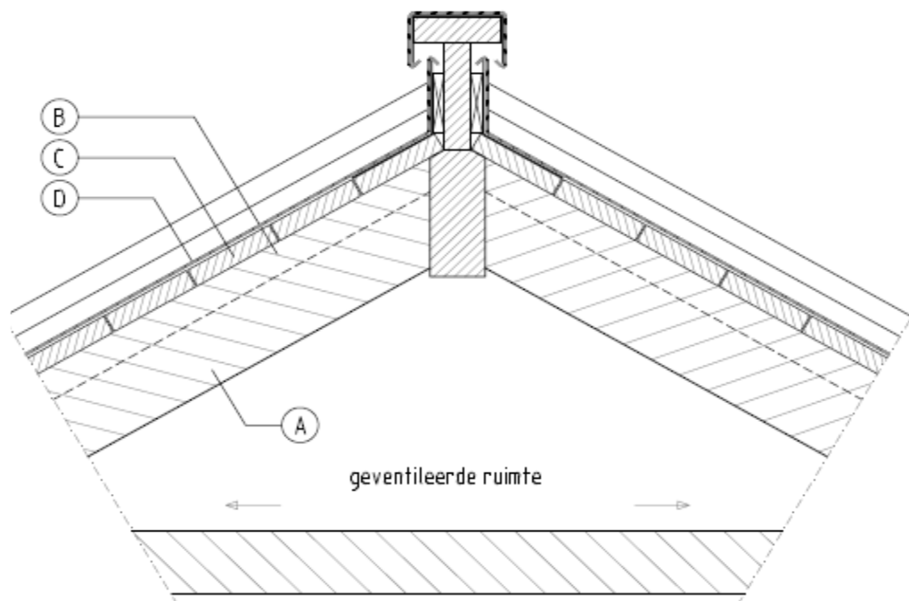
Afb. 27 ongeventileerde nok
