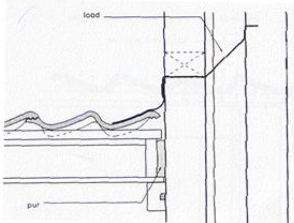
Afb. 51 Zij-aansluiting loodstrook
